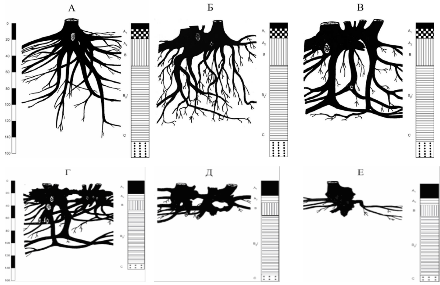
Рис. 2. Строение корневой системы дуба скального семенного (А) и вегетационного происхождения первого (Б), второго (В), третьего (Г), четвертого (Д) и пятого (Е) поколения
